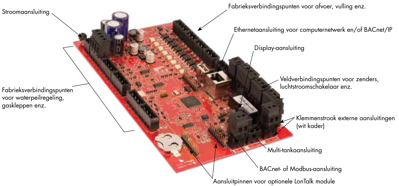
AFBEELDING 4-1: VAPOR-LOGIC PRINTPLAAT
