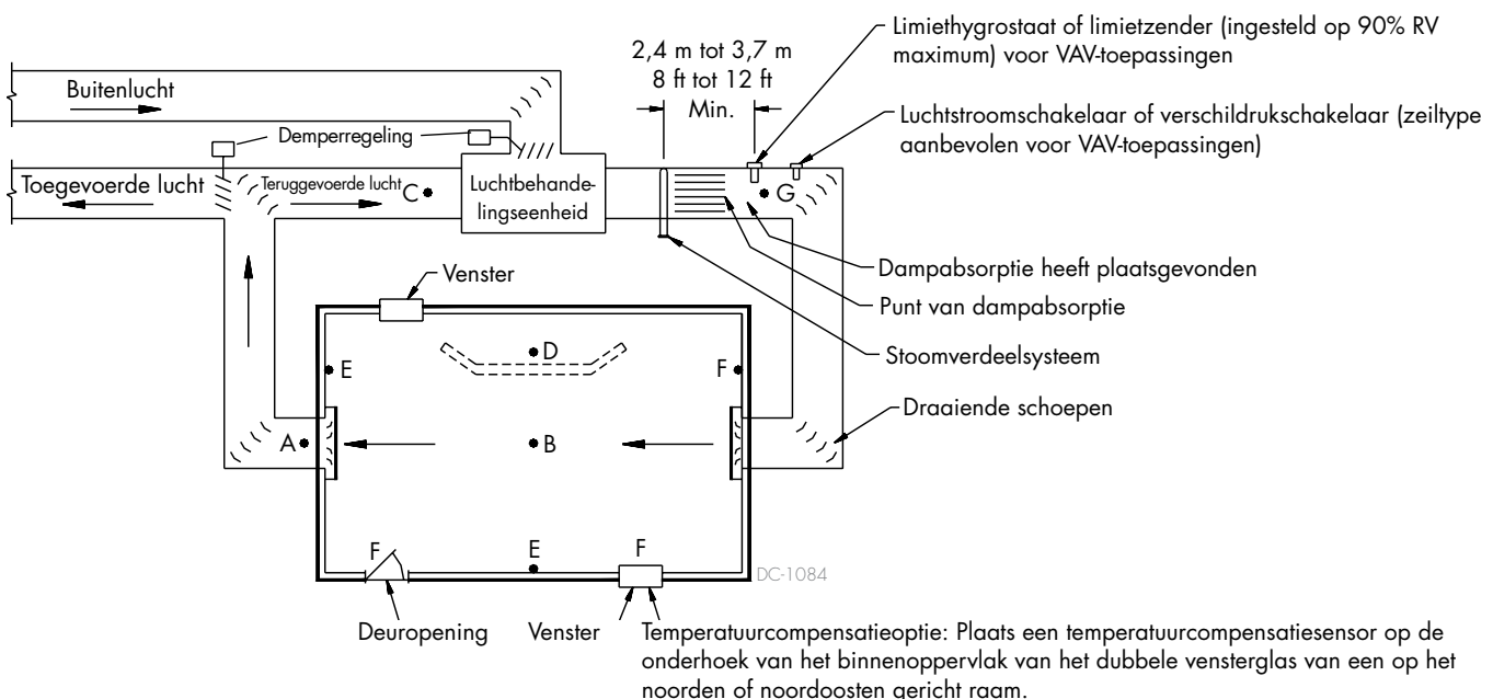
AFBEELDING26-1: AANBEVOLEN SENSORLOCATIE
